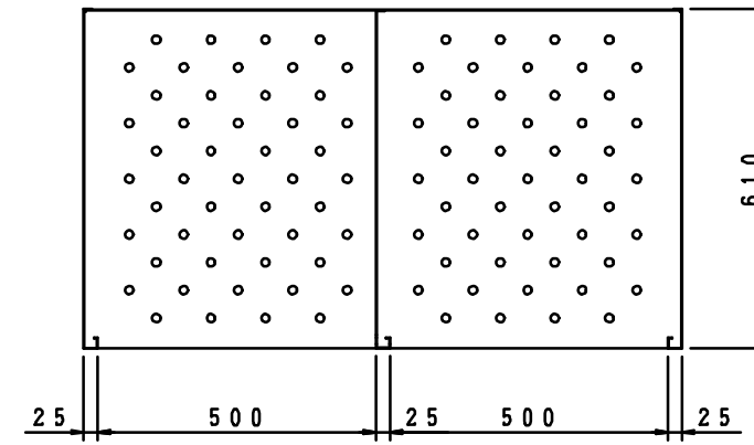
下段収納庫本体横断面
