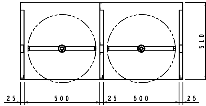
防火衣収納庫本体横断面
