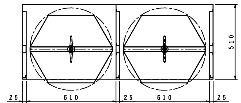
防火衣収納庫本体横断面
