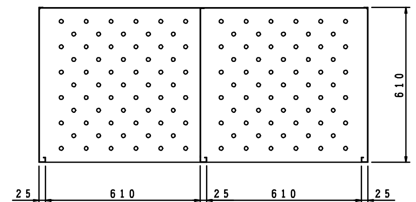
下段収納庫本体横断面
